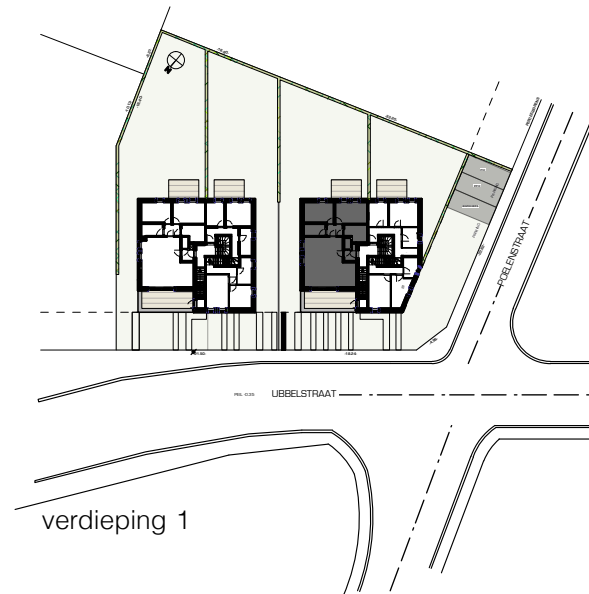
INPLANTINGSPLAN_nieuwe toestand SCHAAL 1/1000
