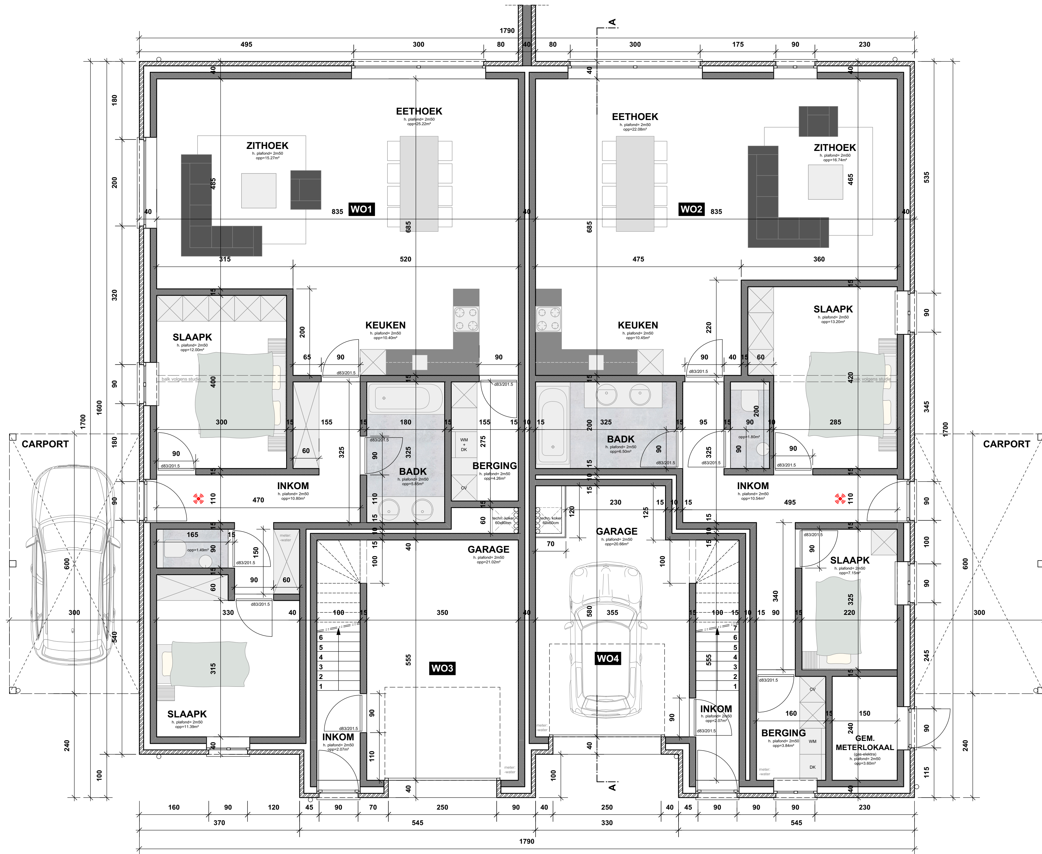
GRONDPLAN nivo +0.00
